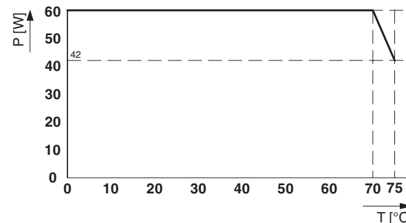
Fig. 6 Derating à partir de 70 °C : 3,6 W/K
