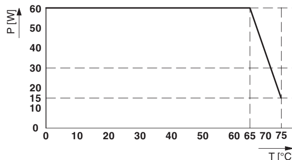
Fig. 7 Derating à partir de 65 °C : 1,5 W/K
