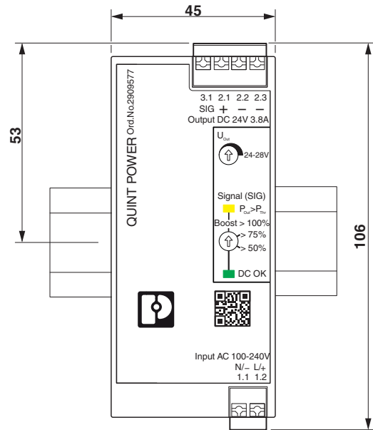
Bild 3 Geräteabmessungen (Maße in mm)
