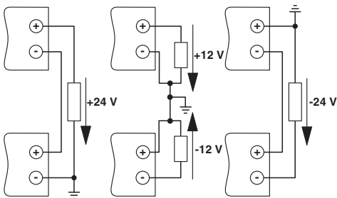
Bild 12 Serieller Betrieb
