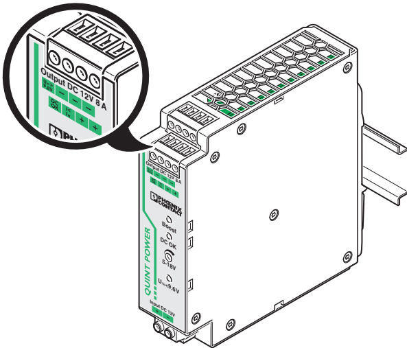
Bild 11 Signalausgänge
