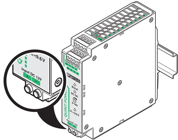
Bild 6 Eingang
