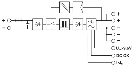
Bild 1 Prinzipschaltbild
