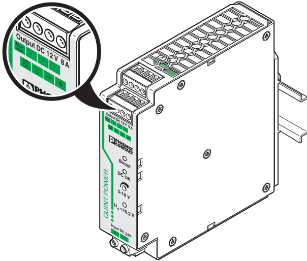
Bild 11 Signalausgänge
