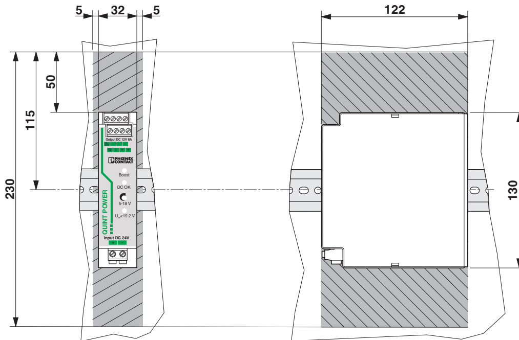
Bild 4 Abmessungen
