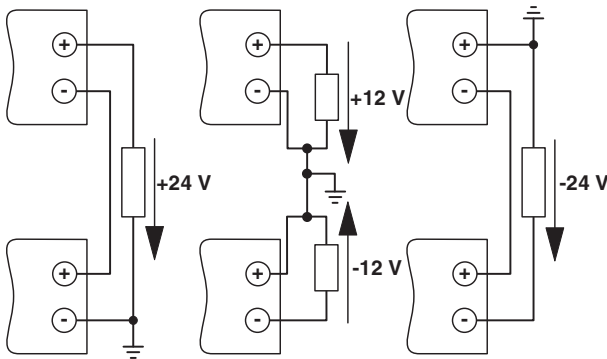
Bild 12 Serieller Betrieb
