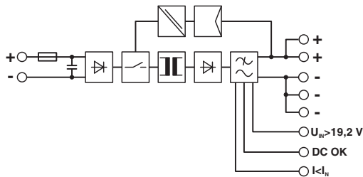
Bild 1 Prinzipaufbau
