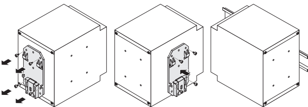
Bild 5 Gedrehte Einbaulage (270° Y-Achse)
