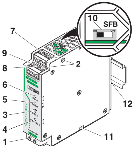
Bild 2 Funktionselemente
