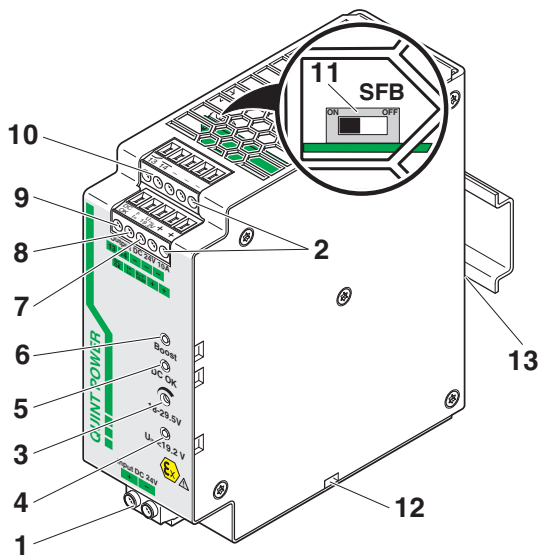
Bild 2 Funktionselemente
