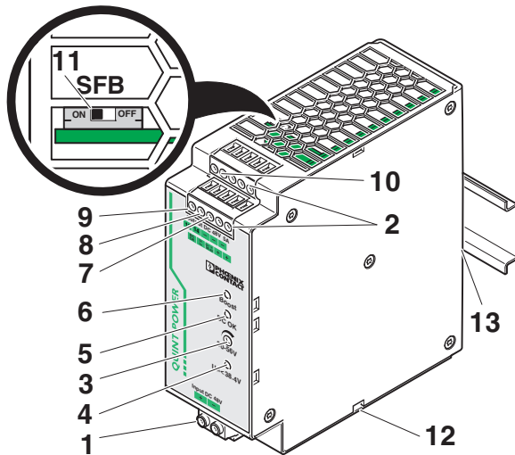
Bild 2 Funktionselemente
