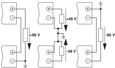
Bild 13 Serieller Betrieb
