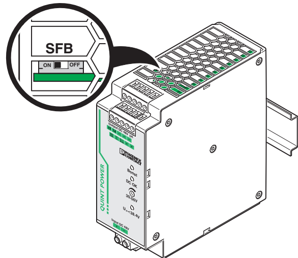
Bild 10 Lage des SFB-Schalters
