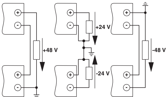
Bild 14 Serieller Betrieb
