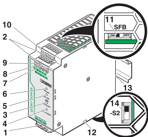
Bild 2 Funktionselemente
