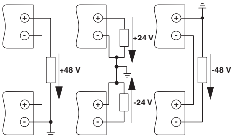
Bild 14 Serieller Betrieb
