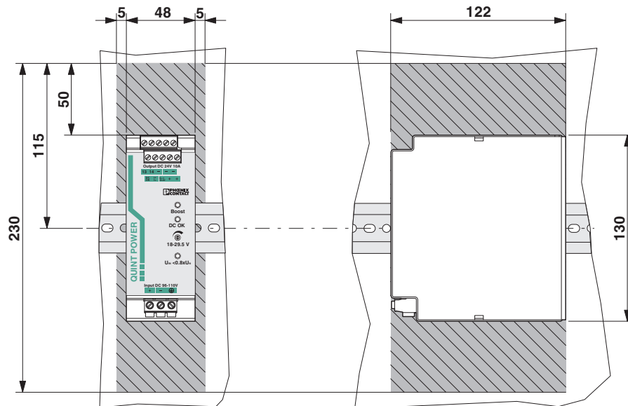
Bild 4 Abmessungen
