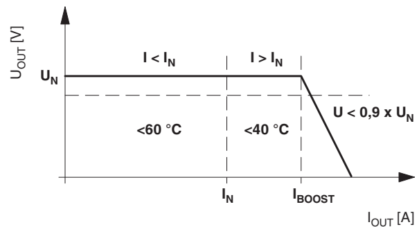
Bild 8 Ausgangskennlinie
