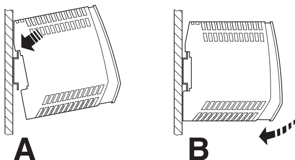
Рисунок 6 Монтаж на несущую рейку
