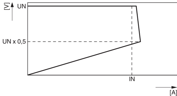
Рисунок 12 Выходная характеристика
