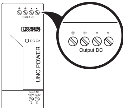
Рисунок 10 Винтовой зажим Output DC +/-
