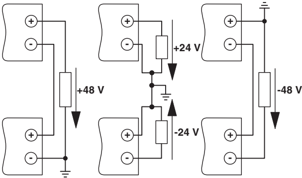
Рисунок 16 Последовательный режим работы
