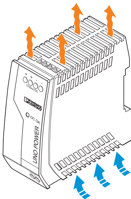
Рисунок 3 Конвекция
