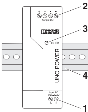
Рисунок 1 Элементы устройств
