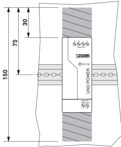
Рисунок 4 Размеры устройства и мертвые зоны
