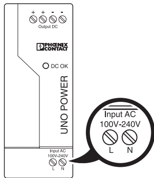
Рисунок 9 Винтовой зажим Input AC L/N
