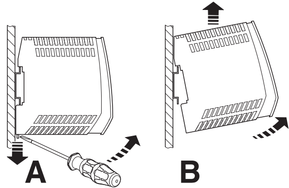
Рисунок 17 Демонтаж
