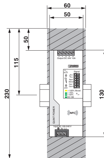
Рисунок 4 Размеры устройства и максимальные закрытые поверхности (мм)
