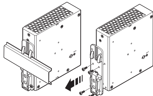
Рисунок 9 Демонтаж универсального адаптера для несущей рейки
