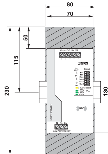
Рисунок 4 Размеры устройства и максимальные закрытые поверхности (мм)
