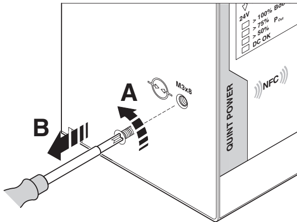
Рисунок 2 Отсоединить газоразрядник
