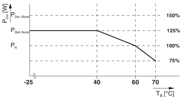
Рисунок 33 Ухудшение характеристик в статическом резерве мощности
