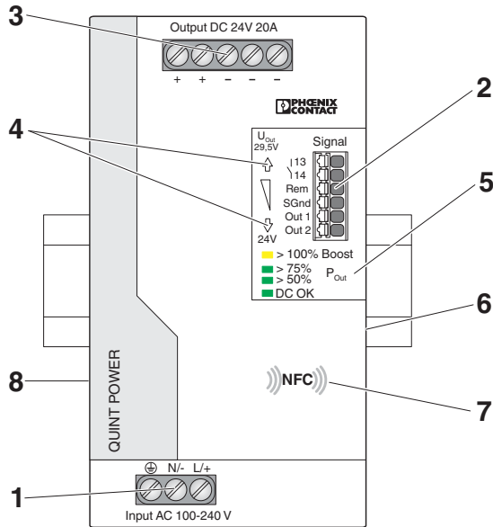
Рисунок 3 Элементы управления и индикации
