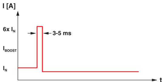
Рисунок 9 Быстрое срабатывание автоматических выключателей благодаря технологии SFB
