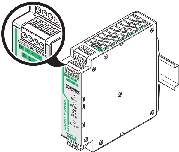
Рисунок 7 Выход
