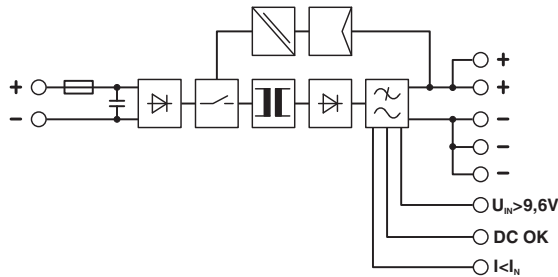
Рисунок 1 Принципиальная схема
