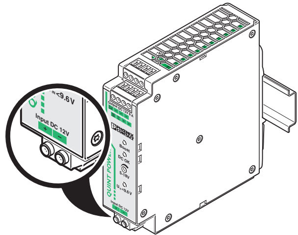
Рисунок 6 вход
