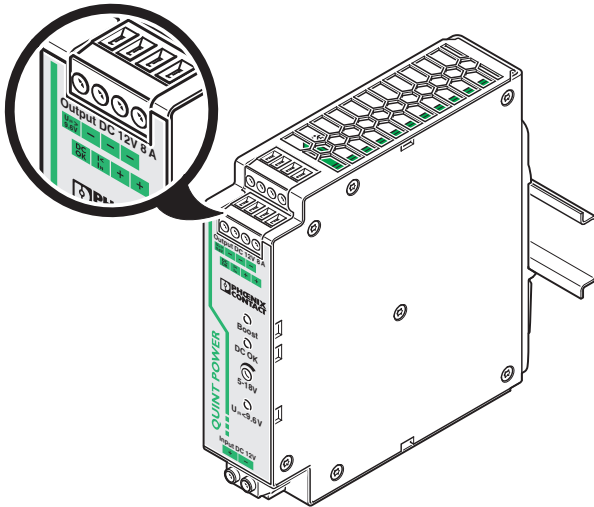
Рисунок 11 Сигнальные выходы
