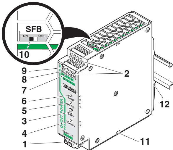
Рисунок 2 Функциональные элементы
