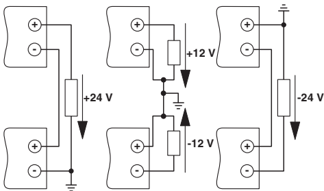
Рисунок 12 Последовательный режим работы
