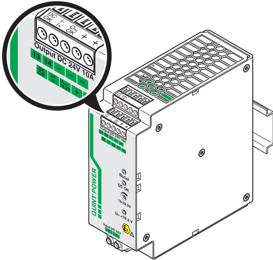
Рисунок 12 Сигнальные выходы
