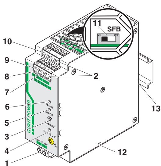
Рисунок 2 Функциональные элементы
