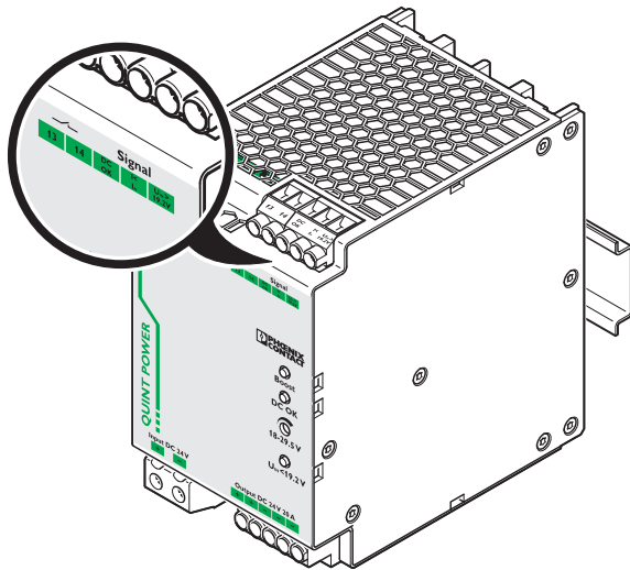
Рисунок 12 Сигнальные выходы
