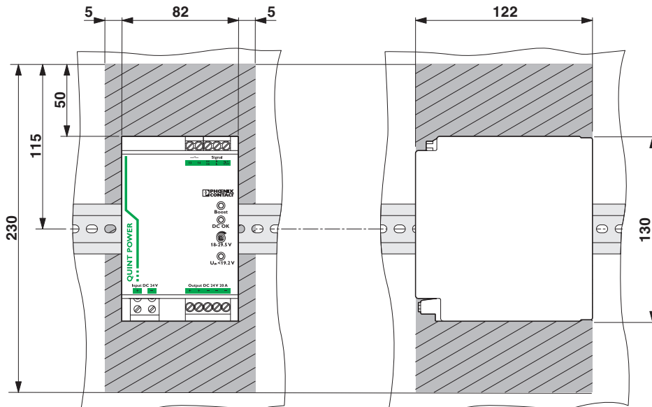
Рисунок 4 Размеры, участки блокировки и положения при встраивании
