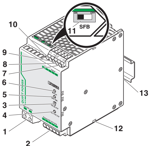
Рисунок 2 Функциональные элементы
