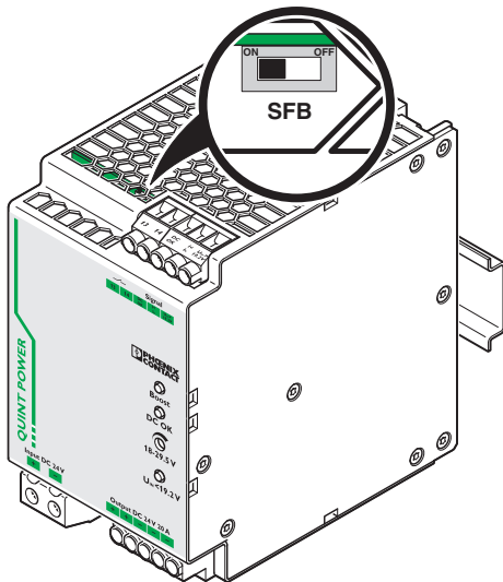
Рисунок 10 Положение переключателя SFB
