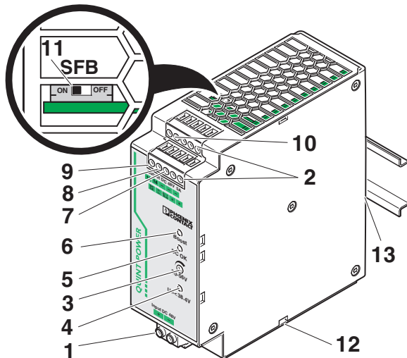
Рисунок 2 Функциональные элементы
