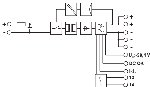
Рисунок 1 Принципиальная схема
