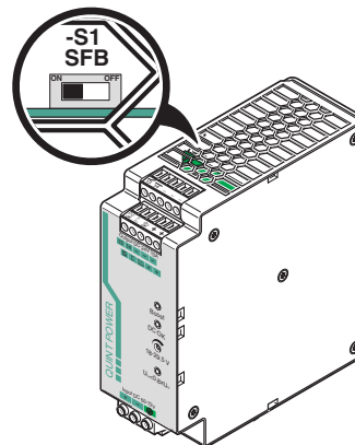
Рисунок 10 Положение переключателя SFB
