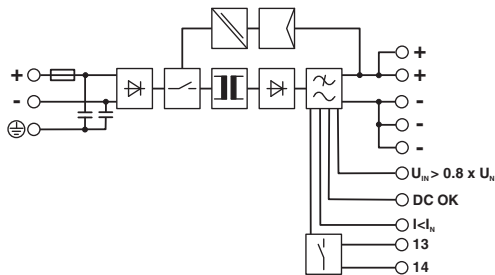
Рисунок 1 Принципиальная схема
