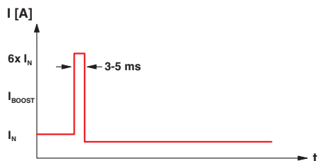
Рисунок 9 Быстрое срабатывание автоматических выключателей благодаря технологии SFB
