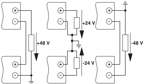
Рисунок 14 Последовательный режим работы
