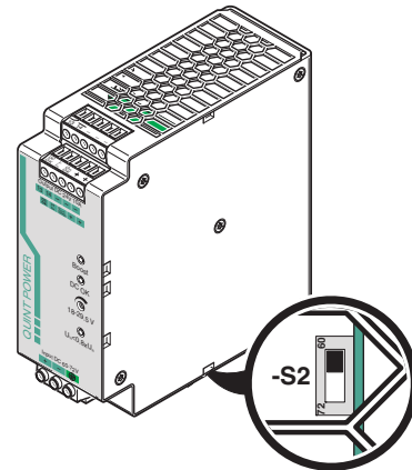
Рисунок 13 Переключатель сигнального порога 60/72 В пост. тока (нижняя часть корпуса)
