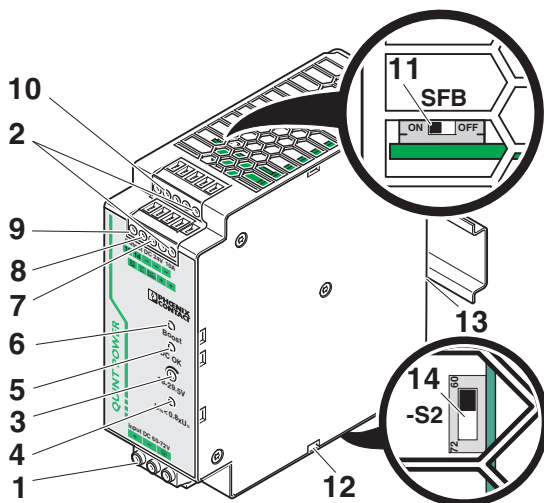
Рисунок 2 Функциональные элементы
