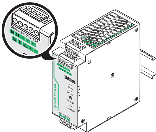
Рисунок 12 Сигнальные выходы
