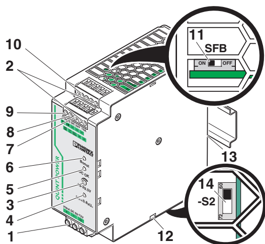
Рисунок 2 Функциональные элементы
