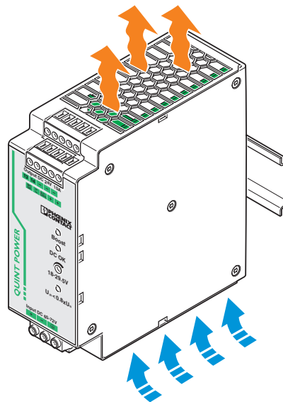
Рисунок 3 Конвекция
