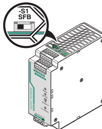
Рисунок 10 Положение переключателя SFB
