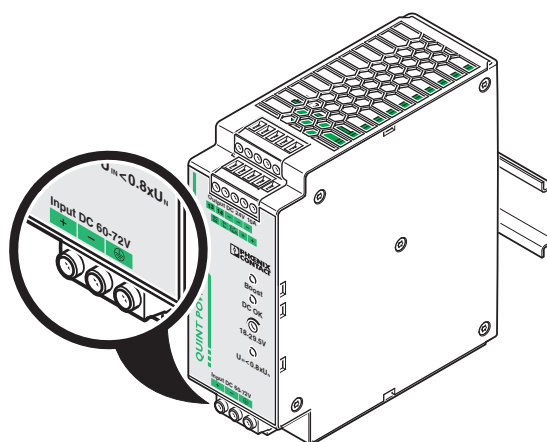
Рисунок 6 вход
