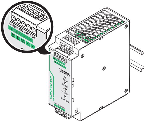
Рисунок 7 Выход
