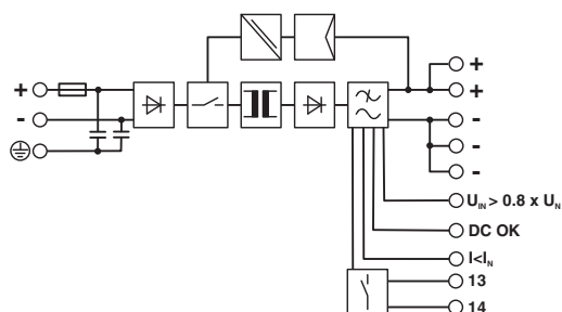
Рисунок 1 Принципиальная схема
