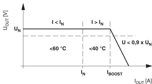
Рисунок 8 Выходная характеристика
