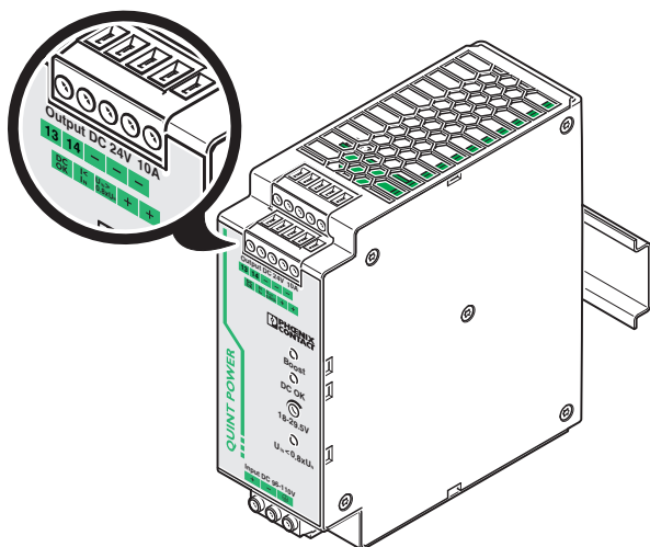
Рисунок 12 Сигнальные выходы
