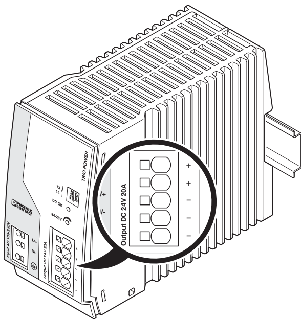
Рисунок 13 Расположение выходных клемм
