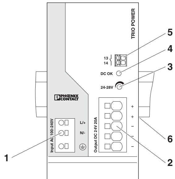
Рисунок 2 Функциональные элементы
