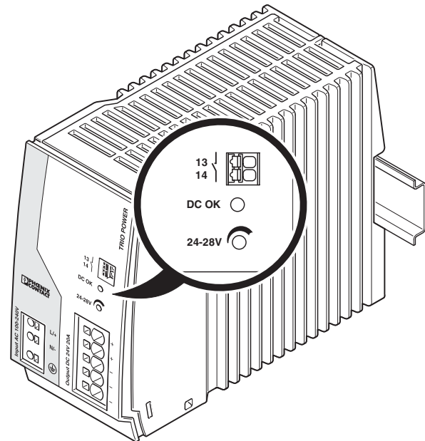
Рисунок 17 Положение элементов
