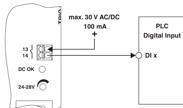
Рисунок 18 Принципиальная схема
