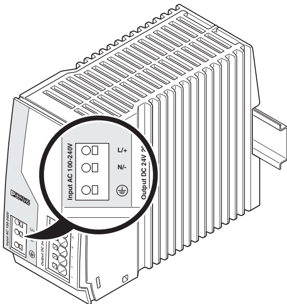
Рисунок 11 Положение входных клемм
