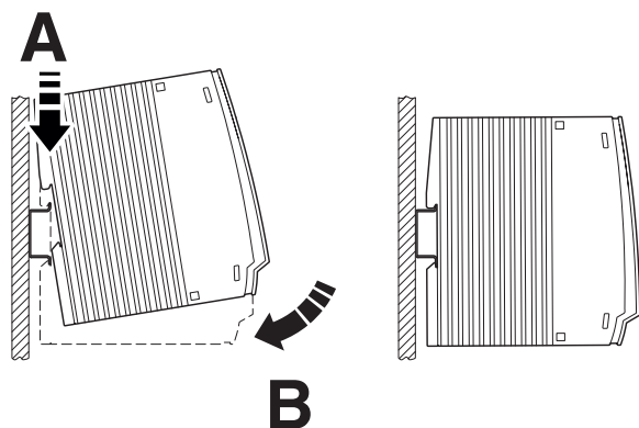
Рисунок 6 Установка на стандартную рейку
