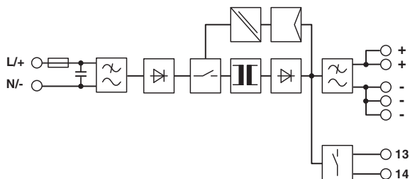
Рисунок 1 Блок-схема
