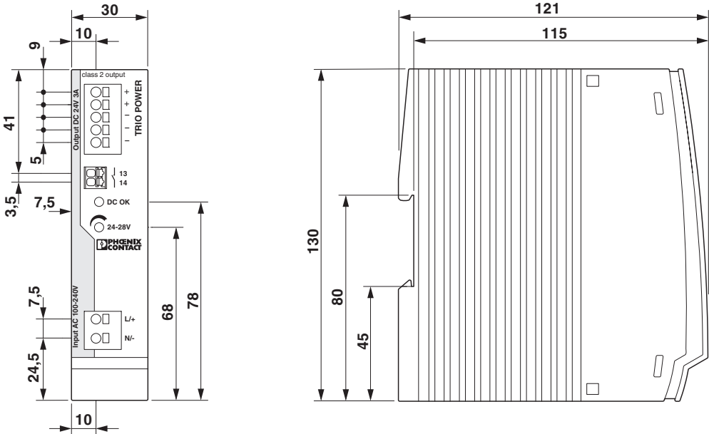
Рисунок 5 Размеры устройства
