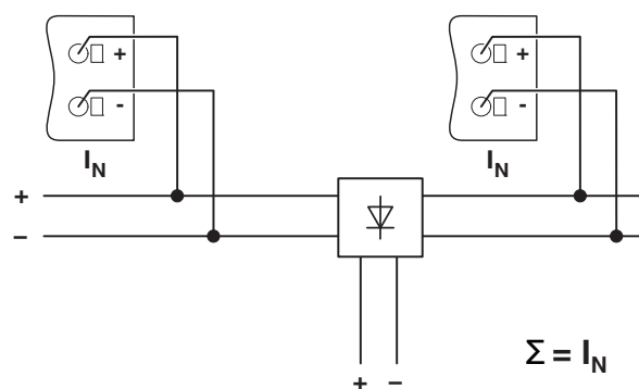
Рисунок 22 Принципиальная схема, развязка через диодный модуль
