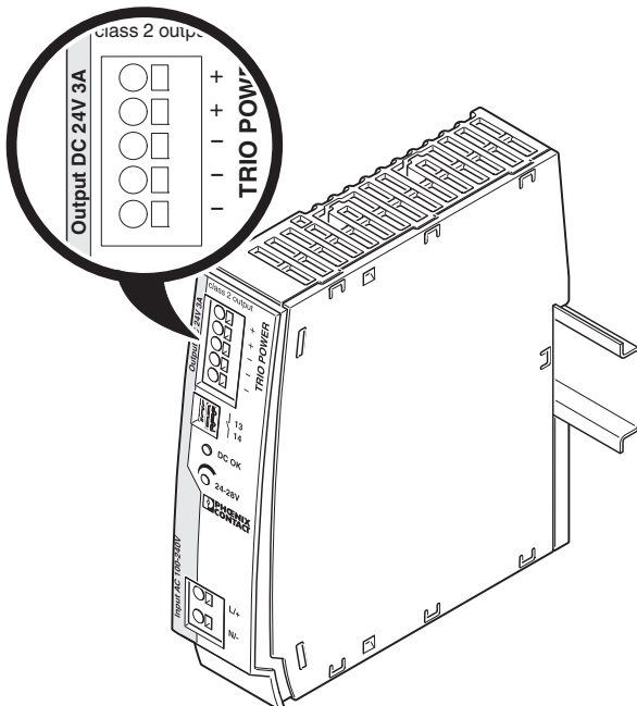
Рисунок 13 Расположение выходных клемм
