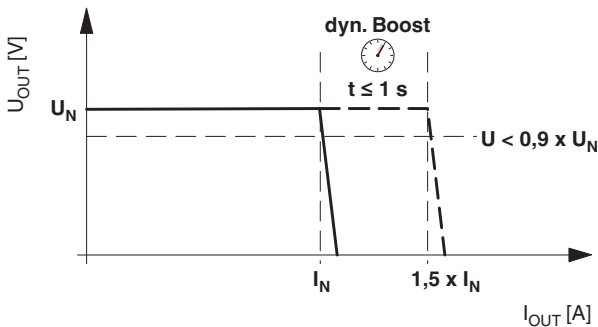
Рисунок 15 Вольтамперная характеристика с динамическим резервом нагрузки
