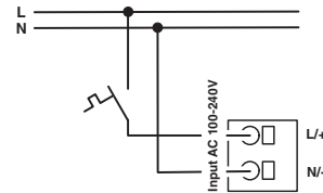
Рисунок 12 Принципиальная схема, подключение входных клемм
