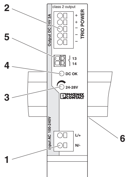
Рисунок 2 Функциональные элементы
