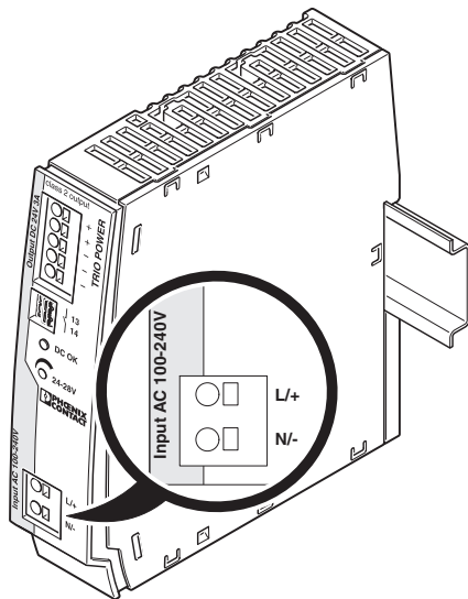
Рисунок 11 Положение входных клемм
