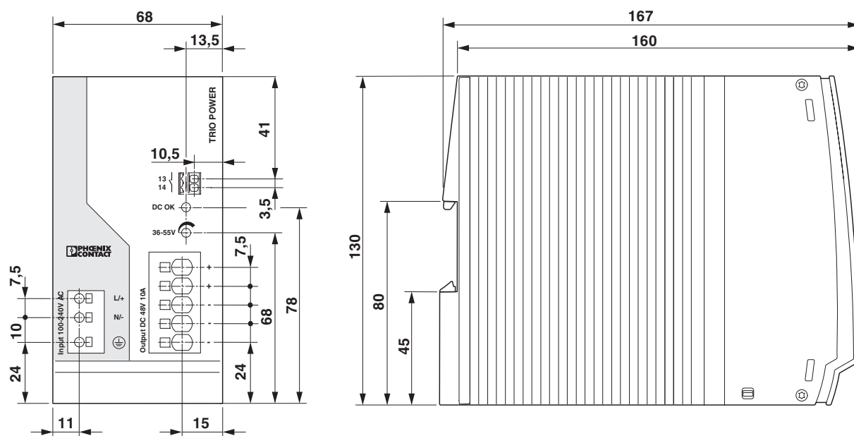
Рисунок 6 Размеры устройства
