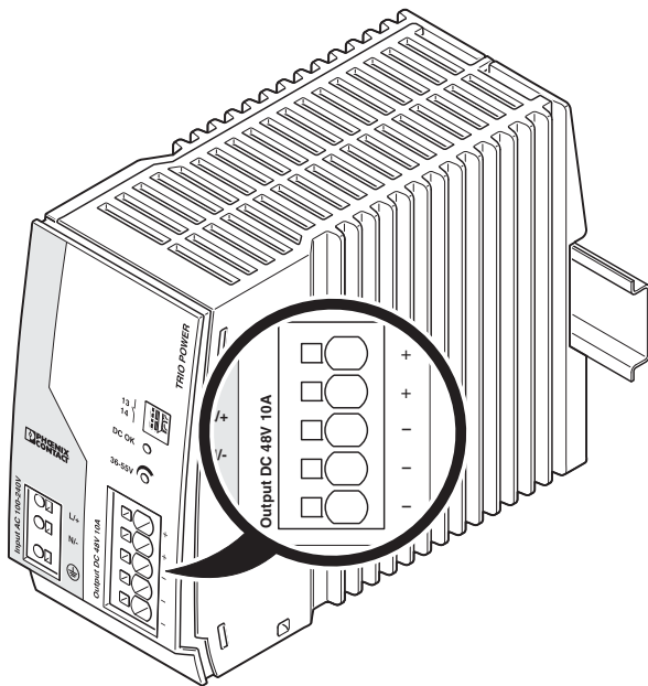
Рисунок 14 Расположение выходных клемм
