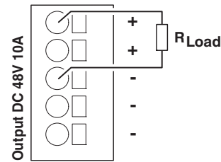
Рисунок 15 Принципиальная схема, подключение выходных клемм
