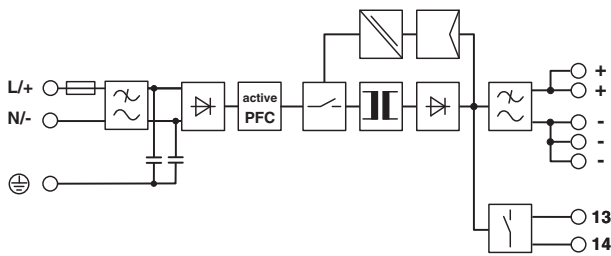
Рисунок 2 Блок-схема
