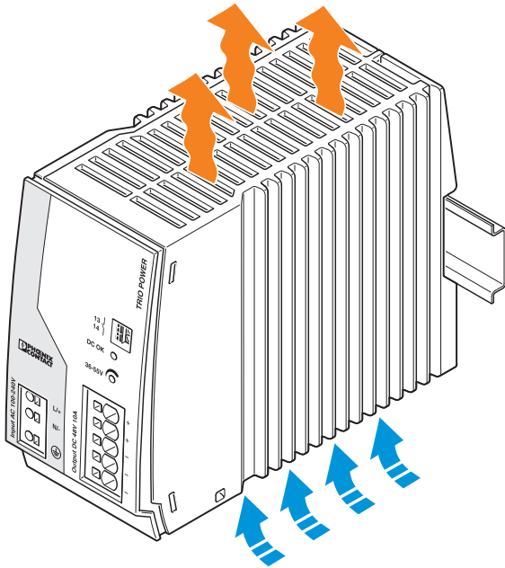
Рисунок 4 Конвекция
