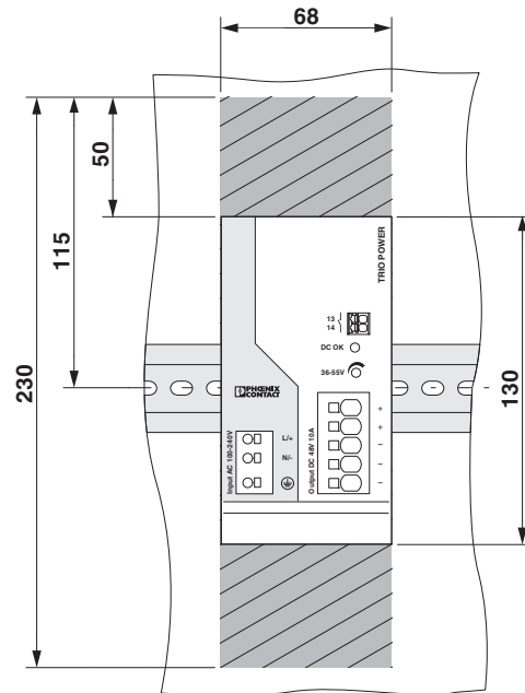
Рисунок 5 Запретные зоны
