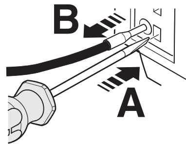
Рисунок 10 Отсоединить кабель (технология подключения Pusch-In)
