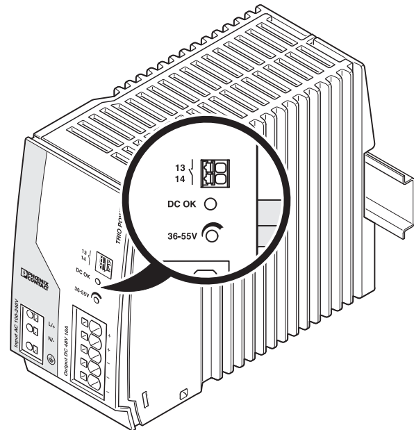
Рисунок 18 Положение элементов
