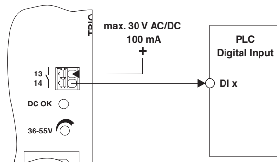
Рисунок 19 Принципиальная схема
