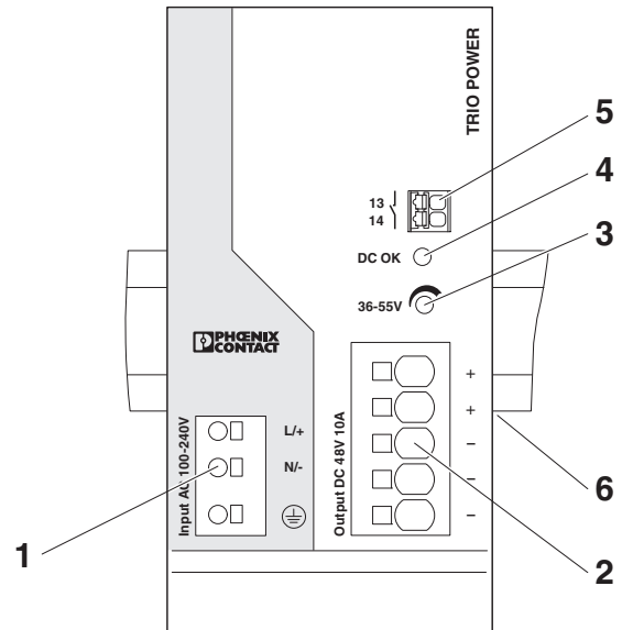
Рисунок 3 Функциональные элементы
