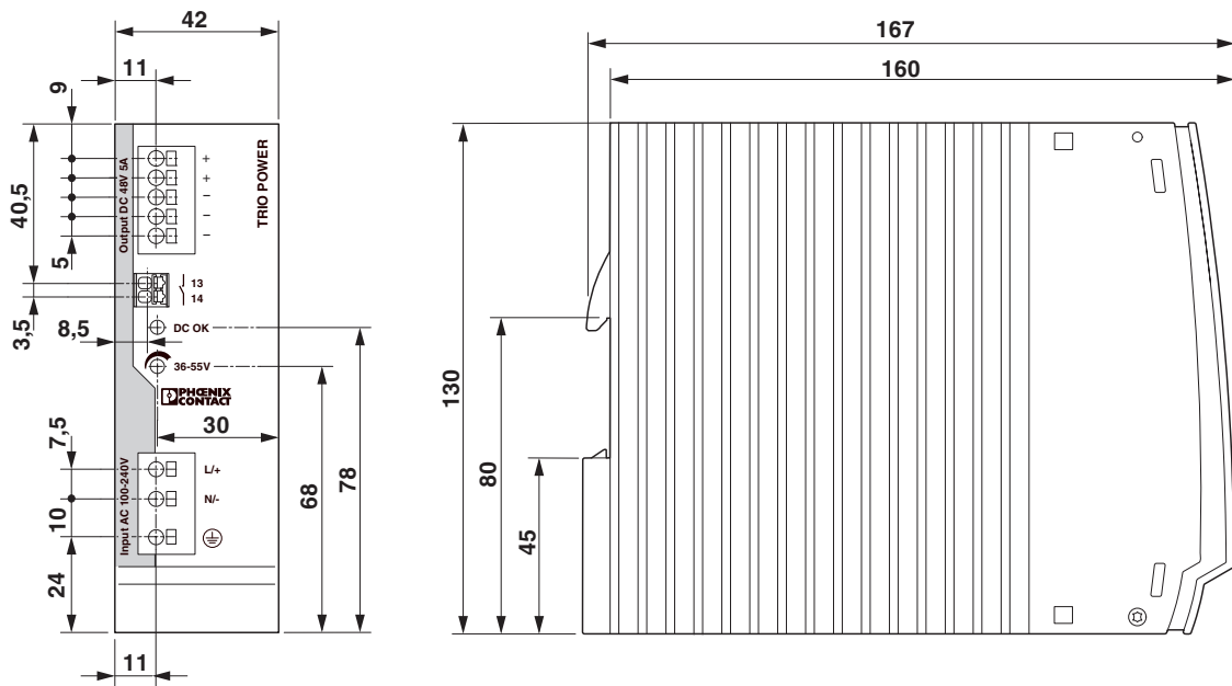
Рисунок 6 Размеры устройства
