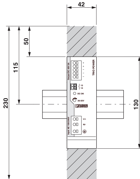
Рисунок 5 Запретные зоны
