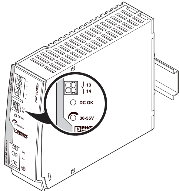
Рисунок 18 Положение элементов
