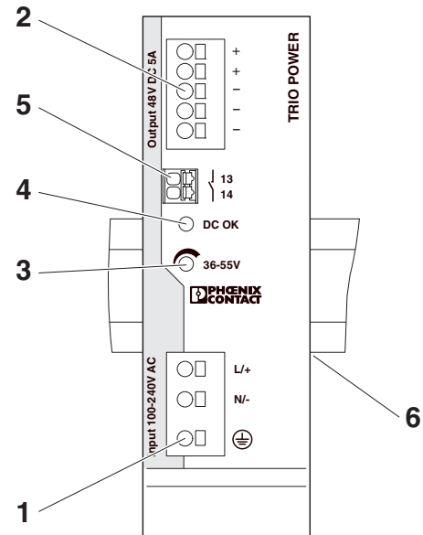
Рисунок 3 Функциональные элементы
