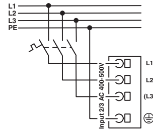
Рисунок 13 Принципиальная схема, подключение входных клемм
