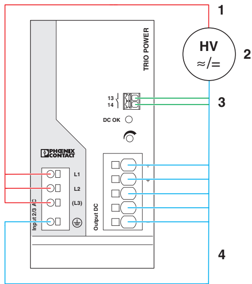
Рисунок 1 Связанная с потенциалом кабельная разводка для испытания высоким напряжением
