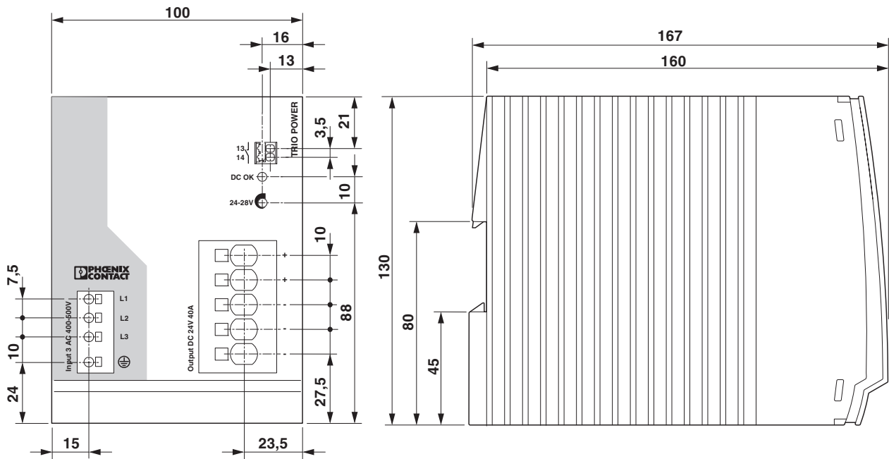
Рисунок 6 Размеры устройства
