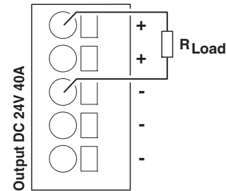
Рисунок 15 Принципиальная схема, подключение выходных клемм
