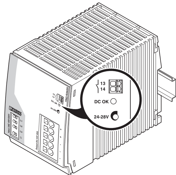
Рисунок 18 Положение элементов
