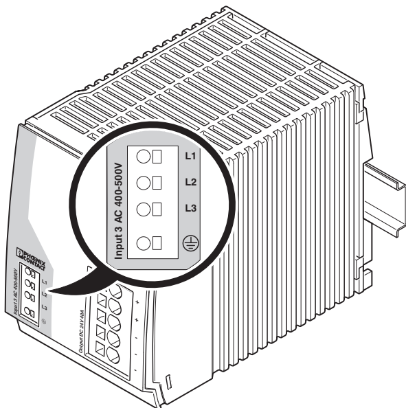
Рисунок 12 Положение входных клемм
