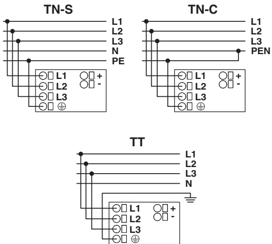
Рисунок 11 Типы сети питания
