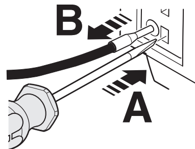
Рисунок 10 Отсоединить кабель (технология подключения Pusch-In)
