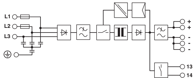
Рисунок 2 Принципиальная схема
