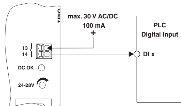
Рисунок 19 Принципиальная схема
