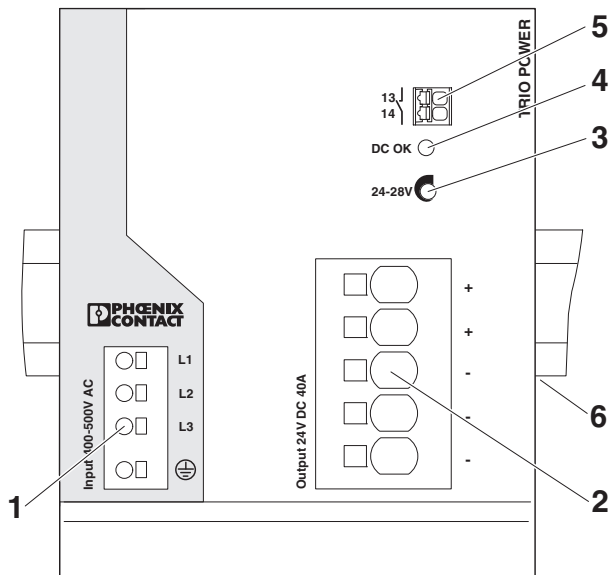
Рисунок 3 Функциональные элементы
