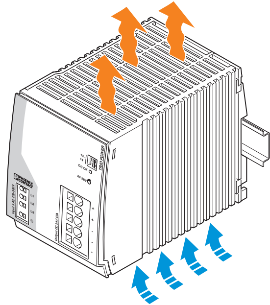
Рисунок 4 Конвекция
