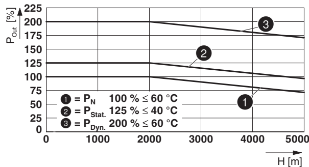
图 34 由海拔高度决定的衰减
