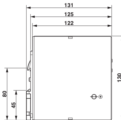
图 5 设备尺寸 (单位 mm)
