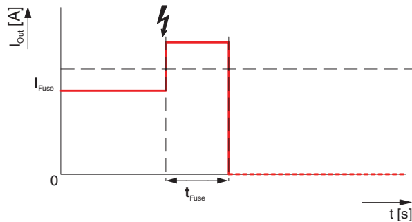
图 18 FUSE MODE 输出特性曲线
