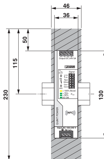
图 4 设备尺寸和最大禁入区域 (单位 mm)
