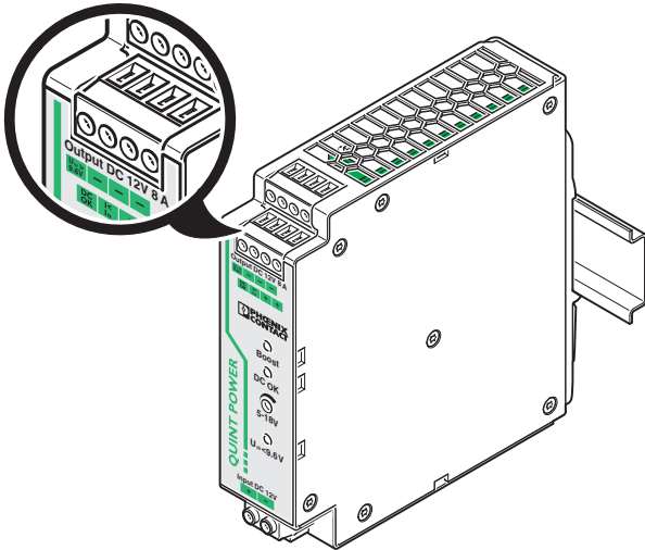
图 7 输出
