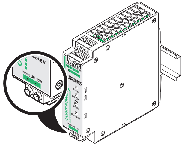
图 6 输入
