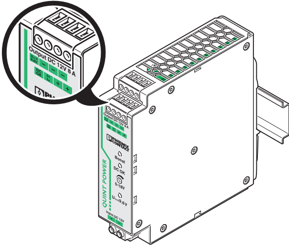
图 11 信号输出
