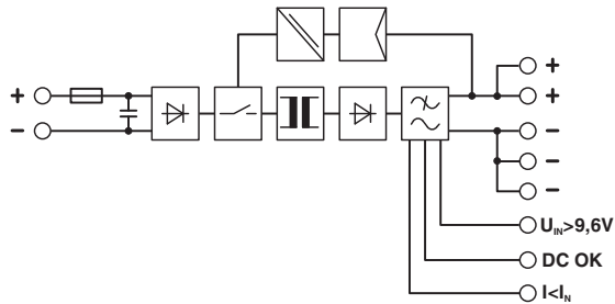
图 1 基本电路图
