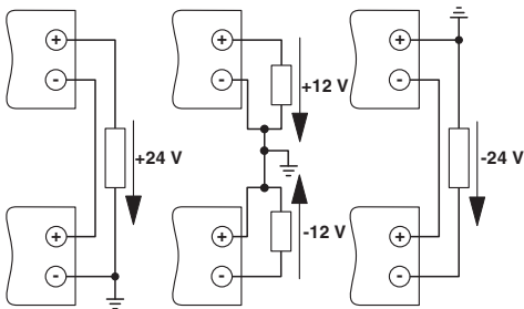
图 12 串联运行
