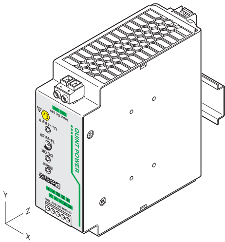
旋转安装位置 (270° X-轴)
