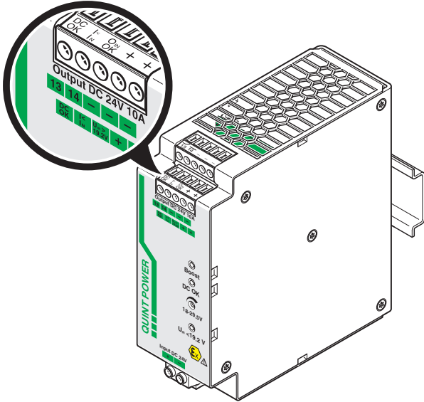
图 12 信号输出
