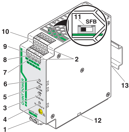
图 2 功能元件
