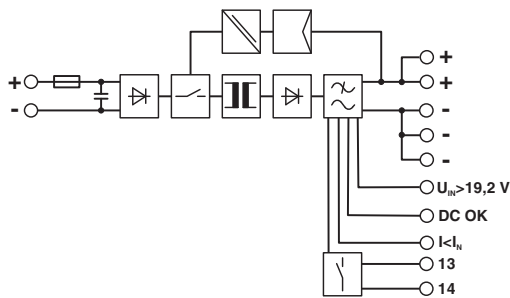
图 1 基本电路图
