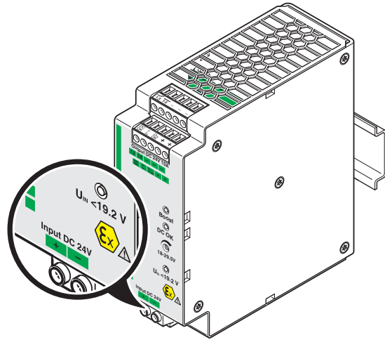
图 6 输入
