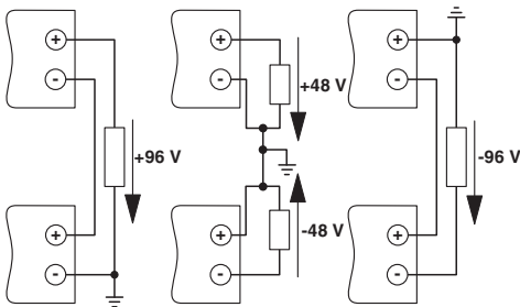
图 13 串联运行
