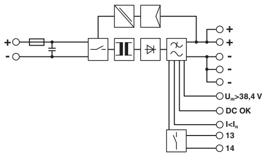
图 1 基本电路图
