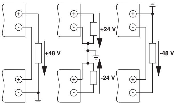
图 14 串联运行
