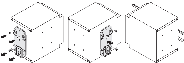
图 5 旋转安装位置 (270° Y 轴)
