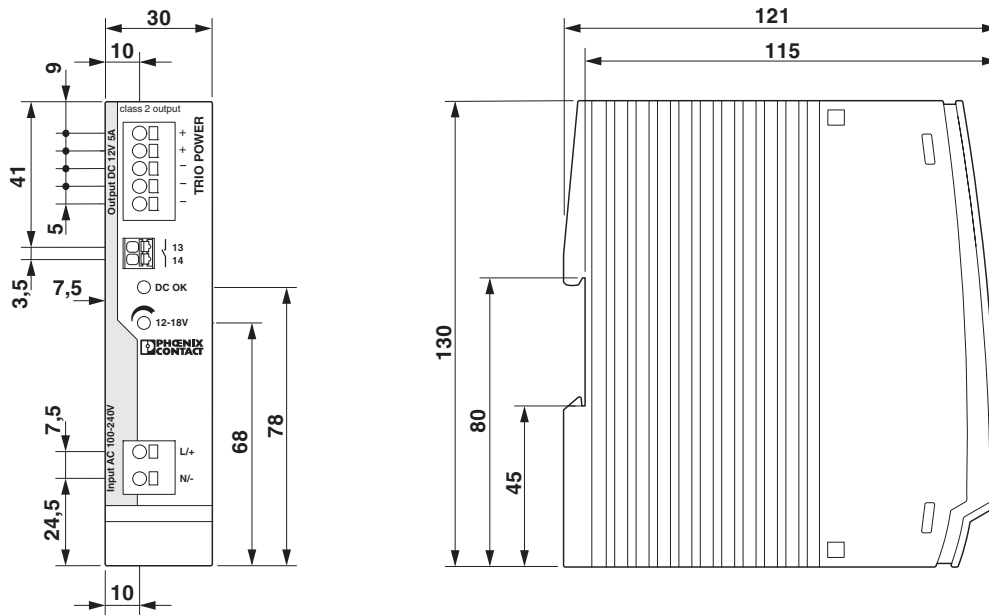
图 6 设备尺寸
