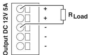
图 15 示意图，切换输出端子
