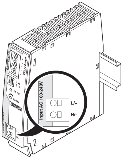
图 12 输入端子位置
