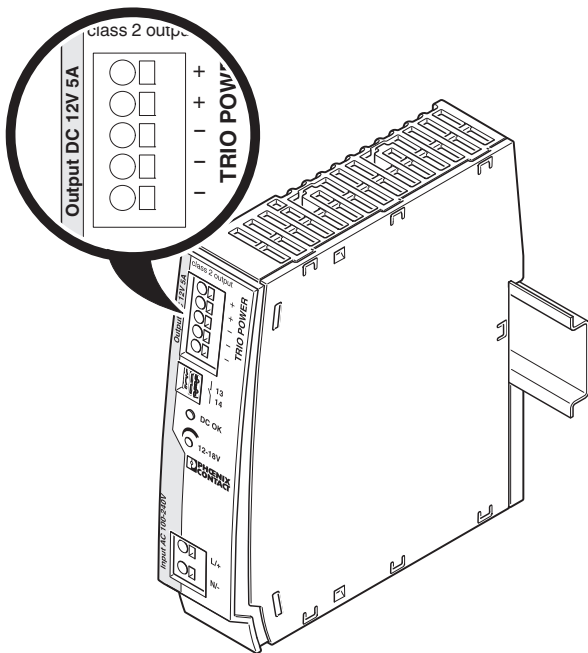
图 14 输出端子位置
