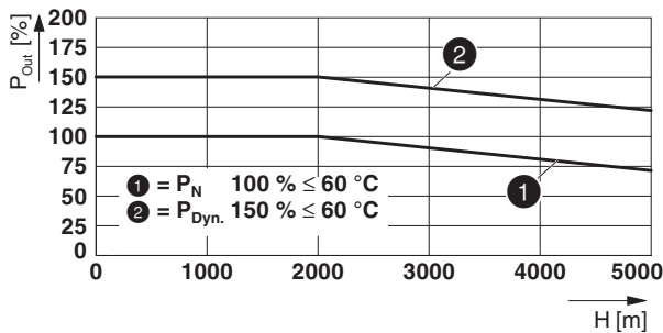
图 20 输出功率取决于安装高度
