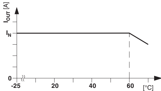
图 19 常规安装位置的温度衰减
