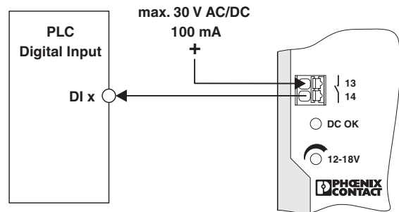
图 18 接线原理
