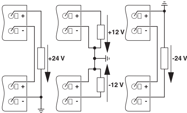
图 21 接线原理，带两个电源时的电压等级
