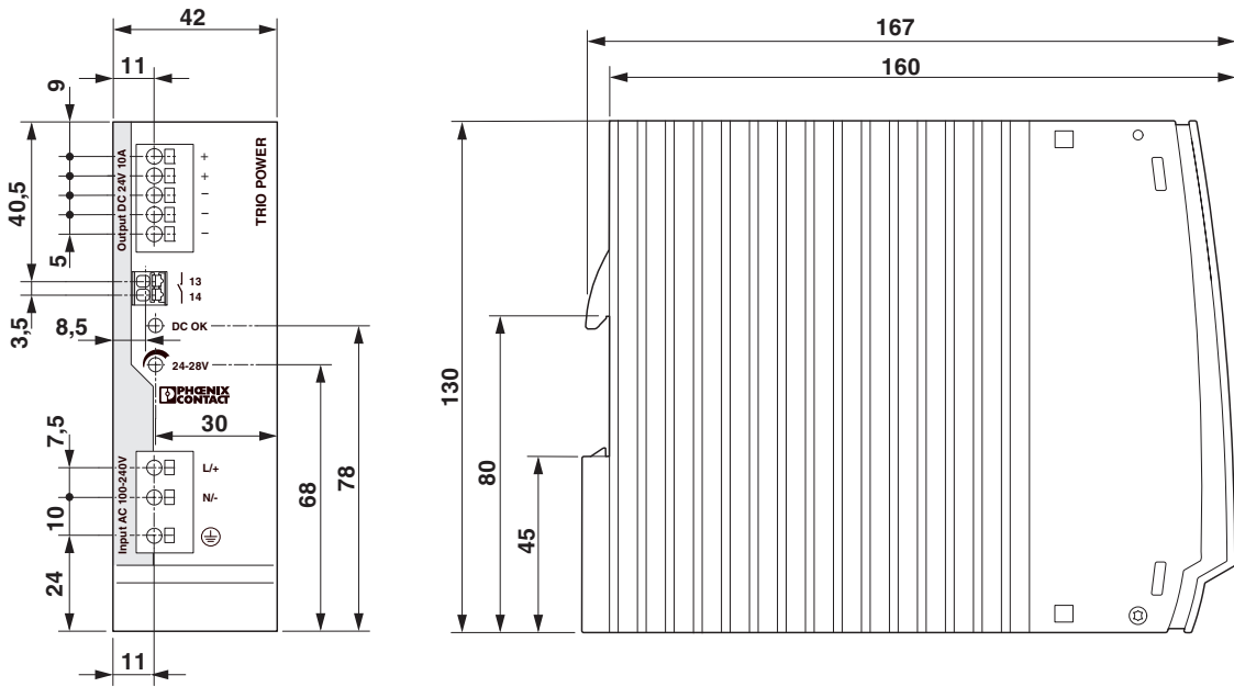
图 5 设备尺寸
