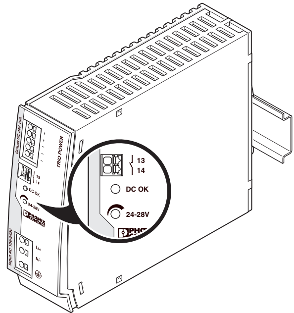
图 17 元件位置
