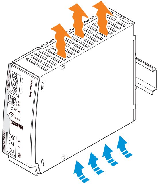
图 3 对流
