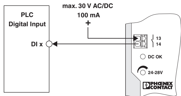
图 18 接线原理
