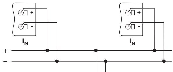
图 26 性能提高的示意图
