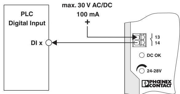
图 19 接线原理
