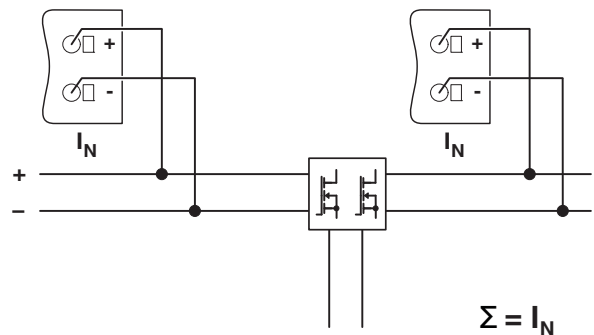
图 25 示意图，通过 ORING 模块解耦
