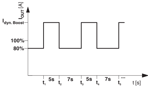
图 17 动态功率增强的示意图
