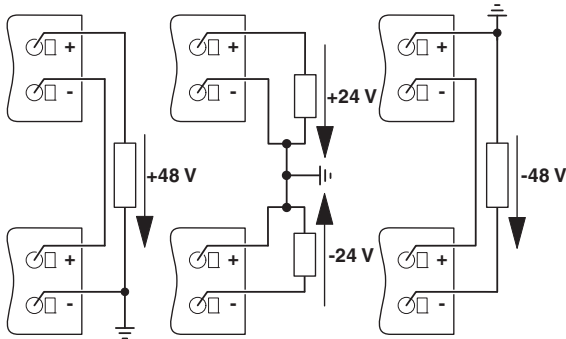
图 22 接线原理，带两个电源时的电压等级
