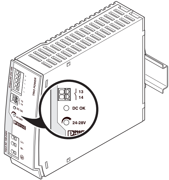
图 18 元件位置
