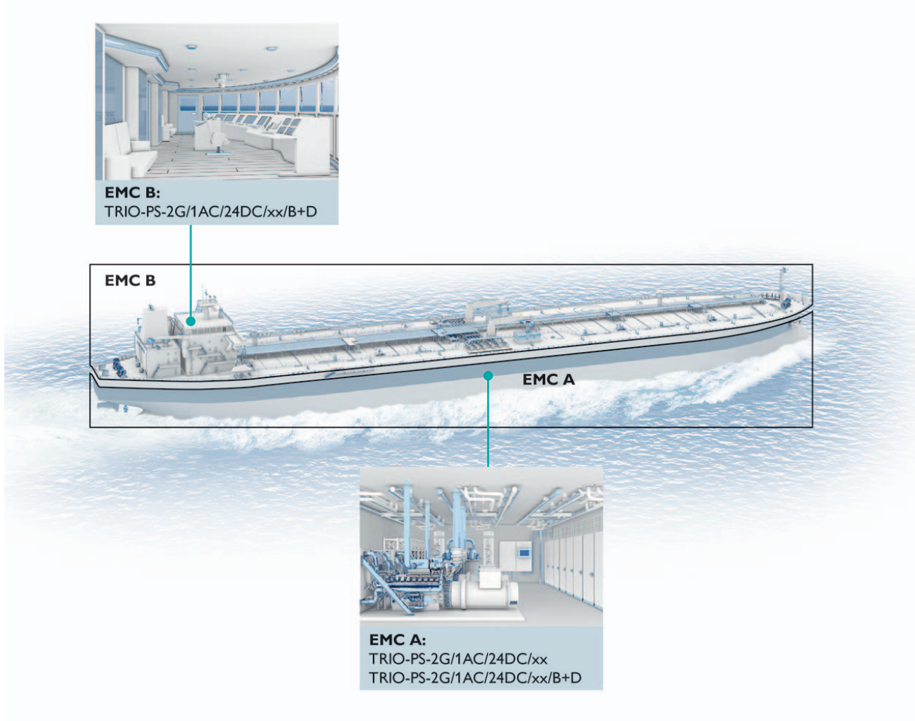
图 27 电磁兼容保护等级的示意图
