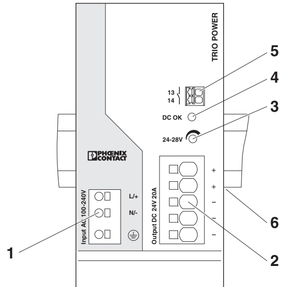
图 2 功能元件
