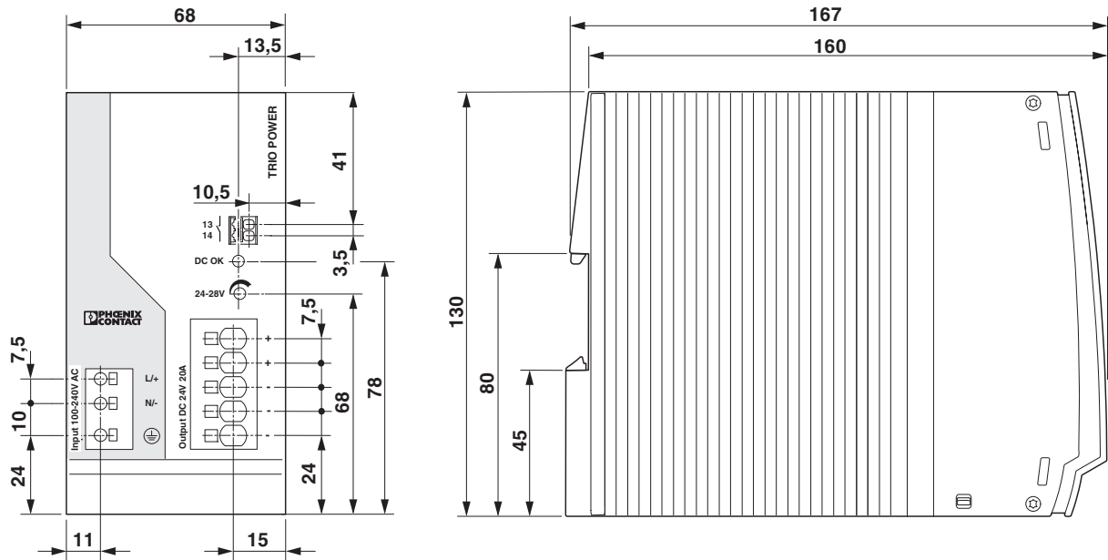
图 5 设备尺寸
