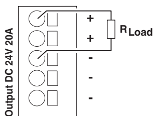
图 14 示意图，切换输出端子
