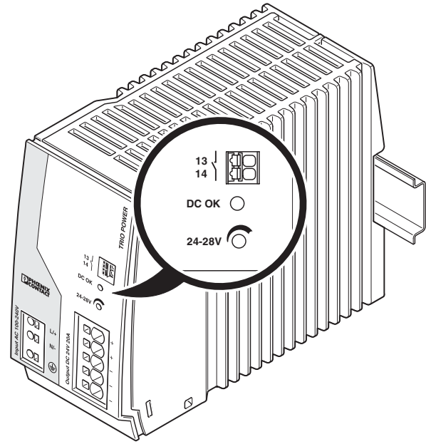
图 17 元件位置
