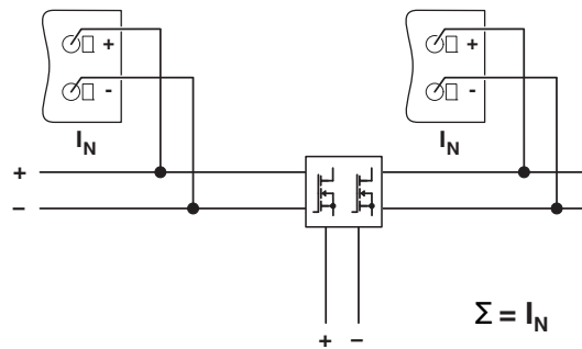
图 23 示意图，通过 ORING 模块解耦
