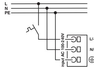
图 12 示意图，切换输入端子
