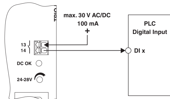
图 18 接线原理
