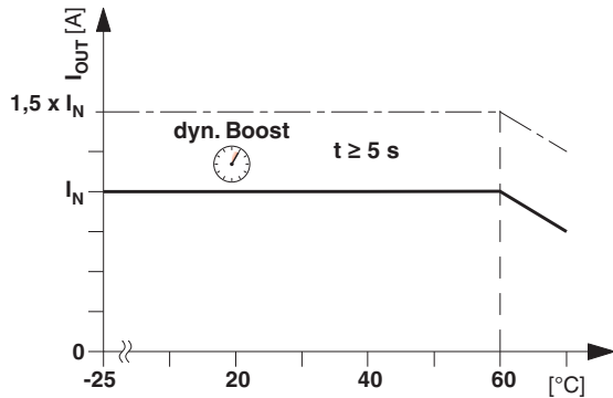
图 19 常规安装位置的温度衰减
