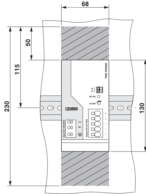
图 4 锁定区域
