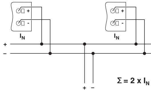
图 24 性能提高的示意图
