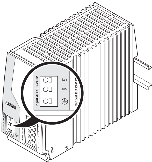
图 11 输入端子位置
