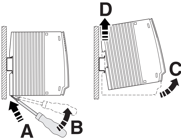
图 7 拆卸 DIN 导轨
