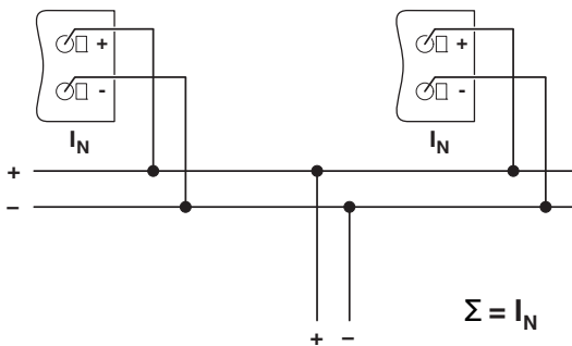
图 21 并行操作示意图
