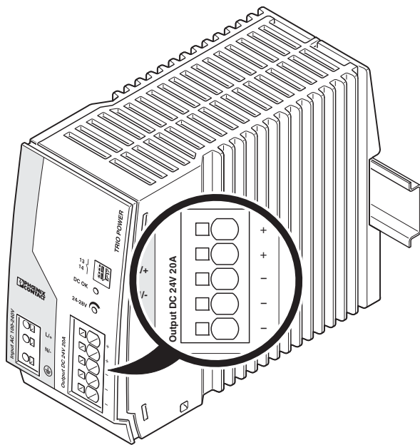
图 13 输出端子位置
