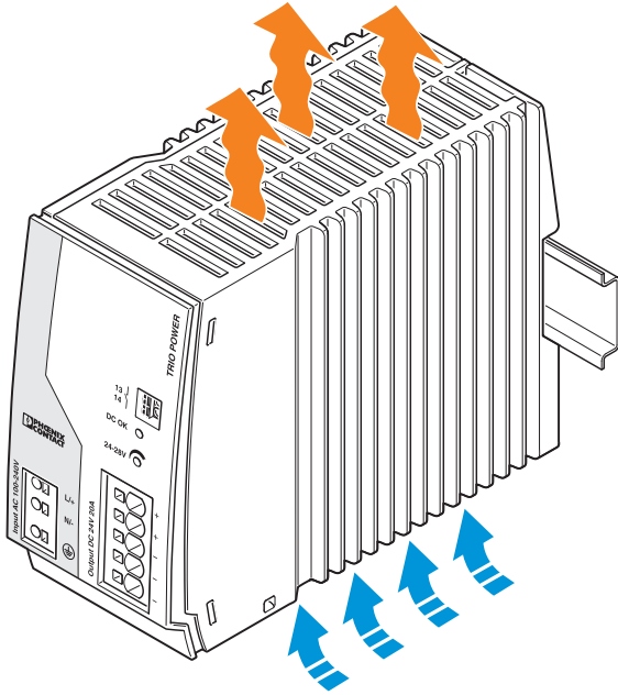
图 3 对流
