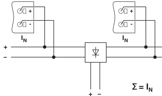
图 22 示意图，通过二极管模块解耦
