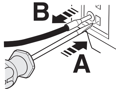
图 9 松开连接电缆（插拔式连接技术）
