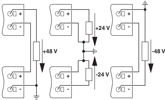
图 20 接线原理，带两个电源时的电压等级
