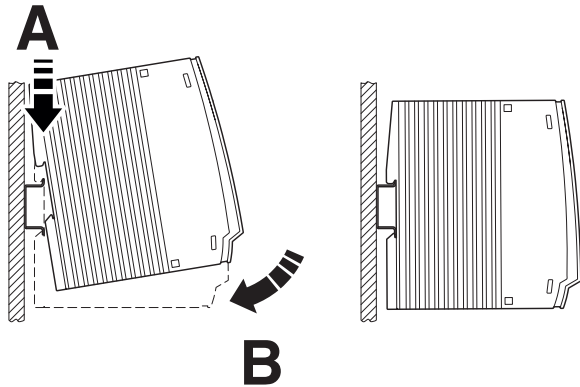
图 6 安装在标准 DIN 导轨上
