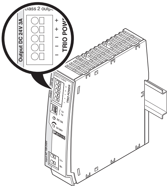
图 13 输出端子位置
