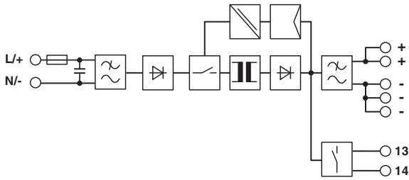
图 1 接线图
