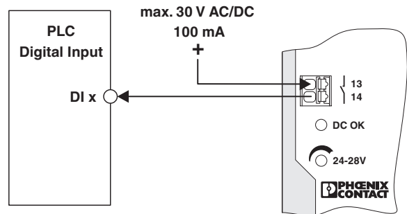
图 18 接线原理
