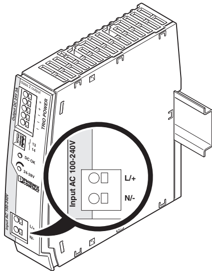
图 11 输入端子位置
