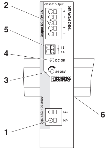
图 2 功能元件
