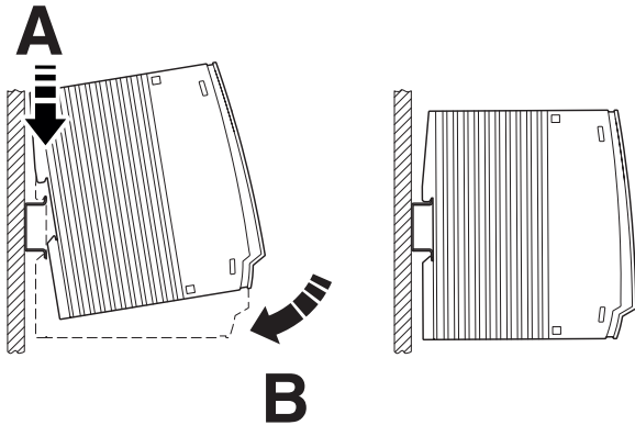
图 6 安装在标准 DIN 导轨上
