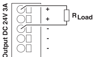
图 14 示意图，切换输出端子
