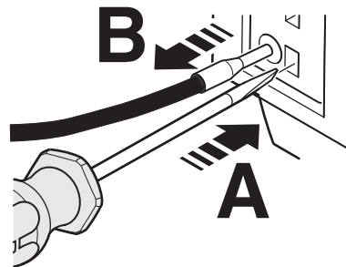
图 9 松开连接电缆（插拔式连接技术）
