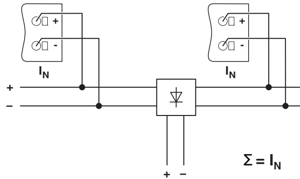
图 22 示意图，通过二极管模块解耦
