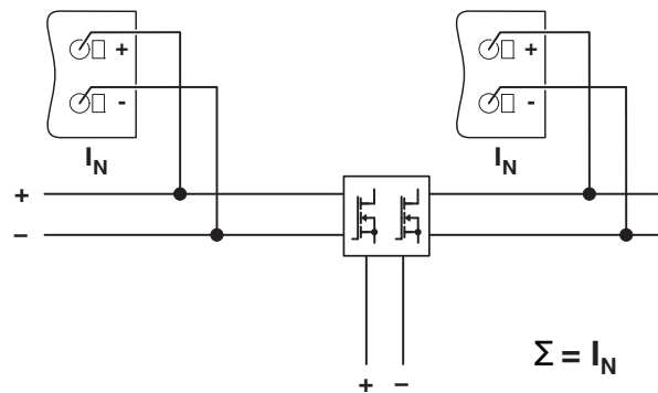
图 23 示意图，通过 ORING 模块解耦
