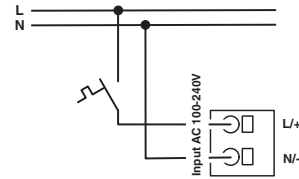
图 12 示意图，切换输入端子
