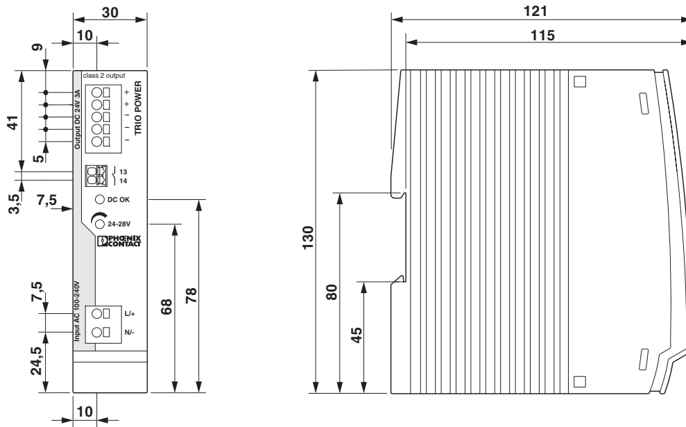
图 5 设备尺寸
