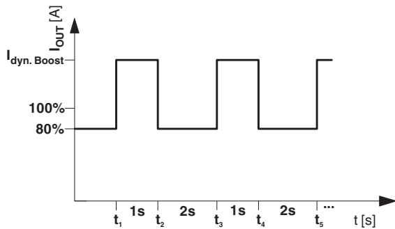
图 16 动态功率增强的示意图
