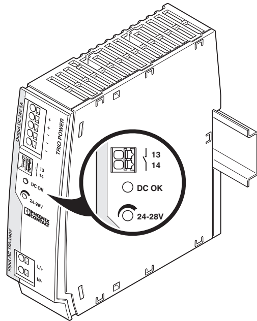
图 17 元件位置
