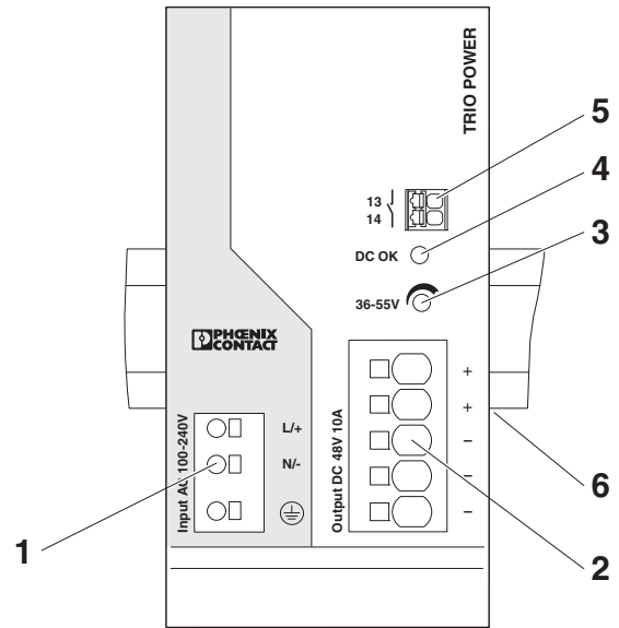
图 3 功能元件
