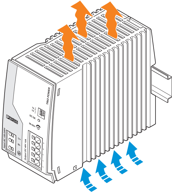
图 4 对流
