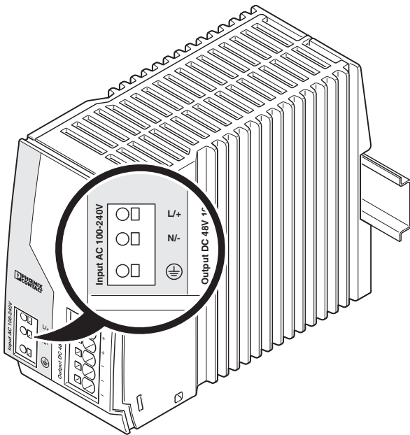
图 12 输入端子位置
