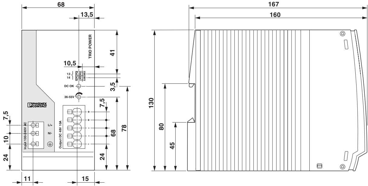
图 6 设备尺寸
