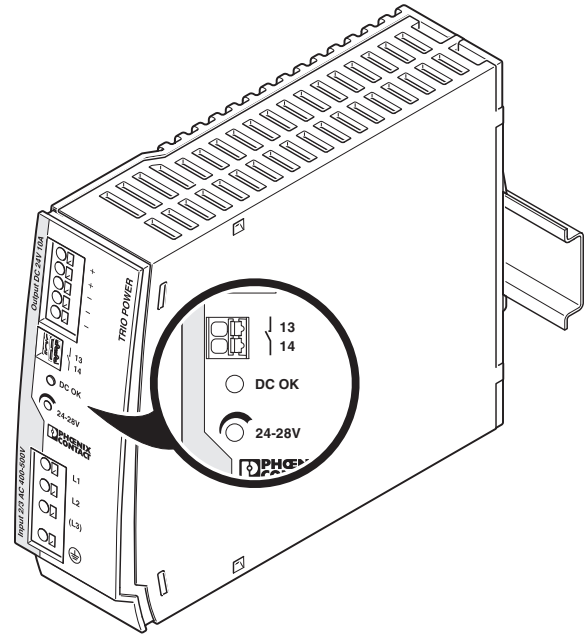
图 17 元件位置
