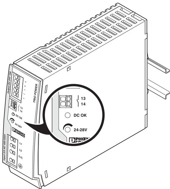
图 13 输出端子位置
