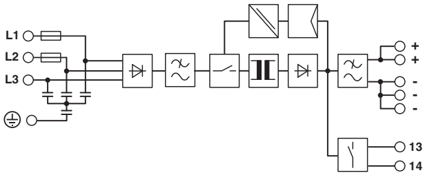
图 1 基本电路图
