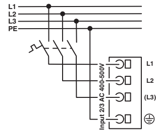
图 12 示意图，切换输入端子
