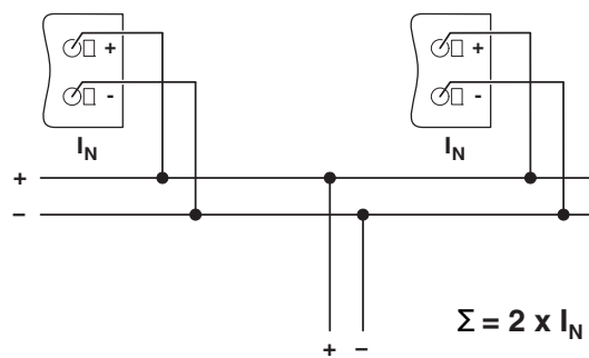
图 24 性能提高的示意图
