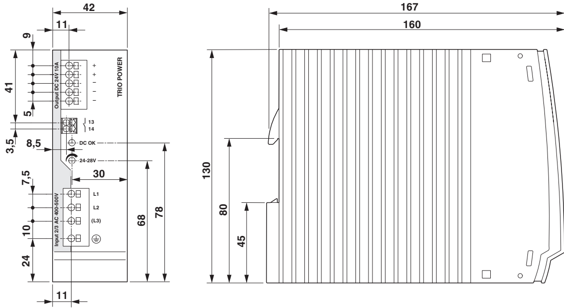
图 5 设备尺寸
