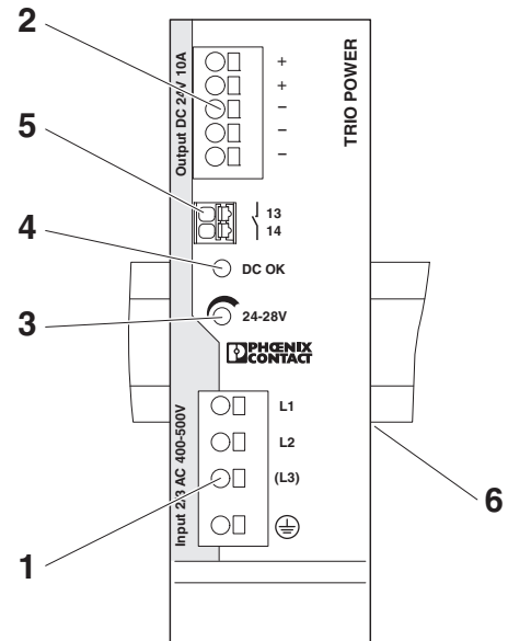
图 2 功能元件
