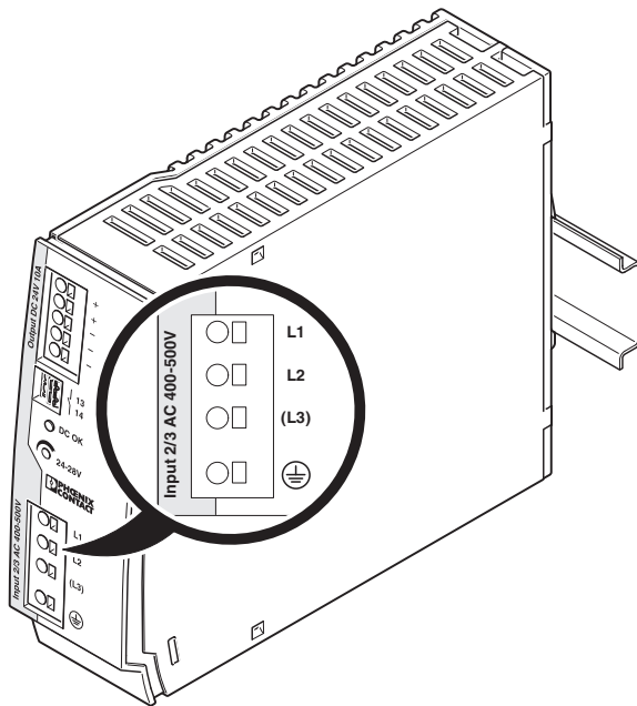
图 11 输入端子位置
