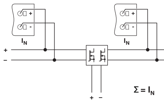
图 23 示意图，通过 ORING 模块解耦
