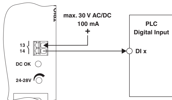
图 18 接线原理
