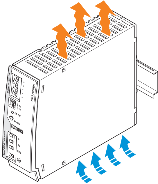
图 3 对流
