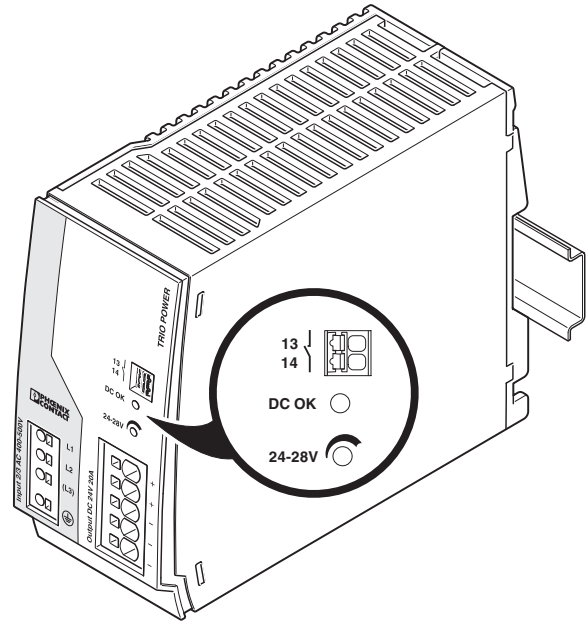
图 17 元件位置
