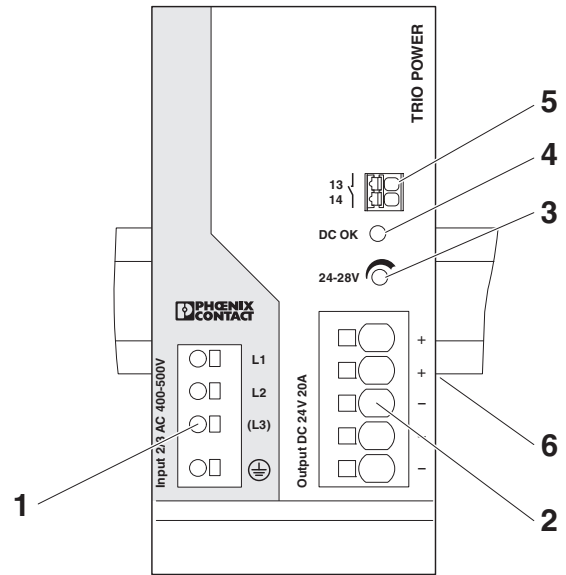
图 2 功能元件
