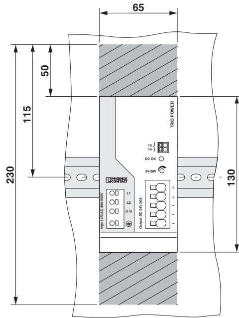
图 4 锁定区域
