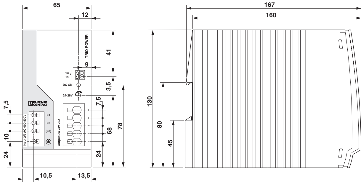
图 5 设备尺寸
