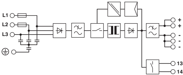
图 2 基本电路图
