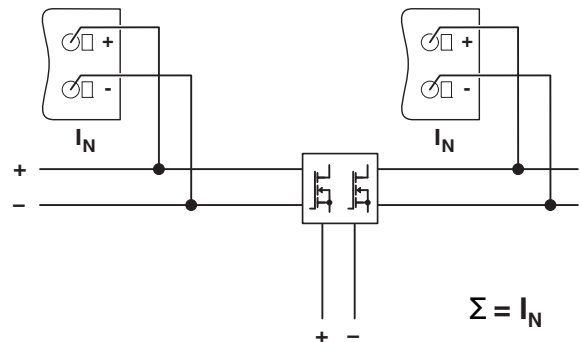
图 25 示意图，通过 ORING 模块解耦
