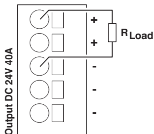
图 15 示意图，切换输出端子
