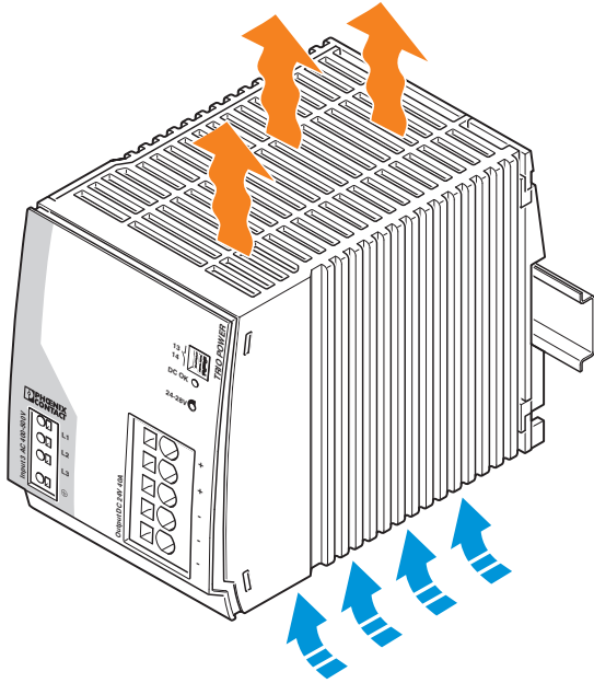
图 4 对流
