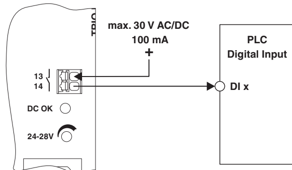
图 19 接线原理
