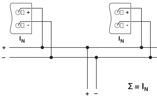
图 23 并行操作示意图
