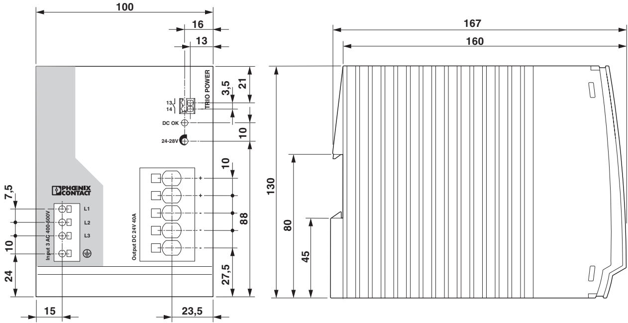
图 6 设备尺寸
