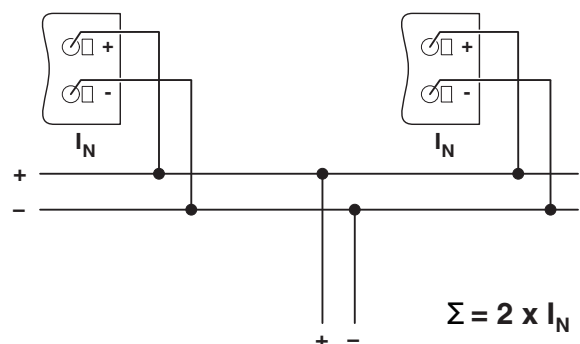
图 26 性能提高的示意图
