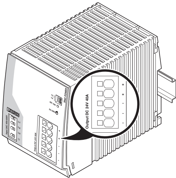
图 14 输出端子位置
