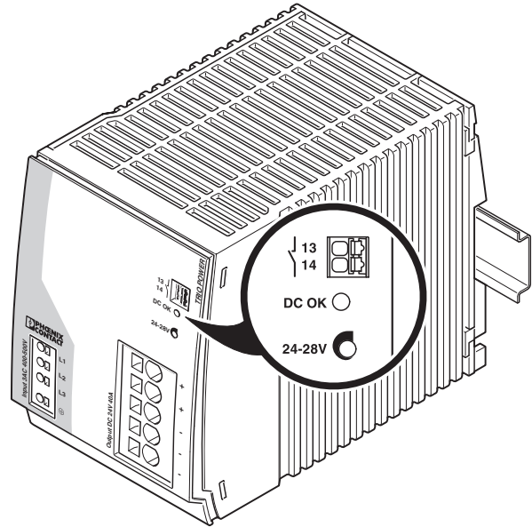
图 18 元件位置
